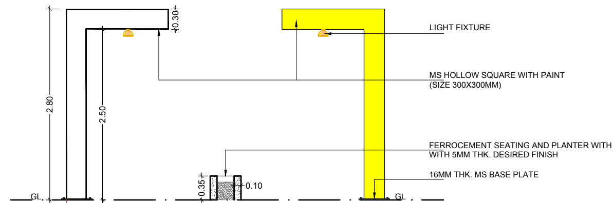
SECTION - 'B-B' (TYP.) (SCALE : 1:50)
