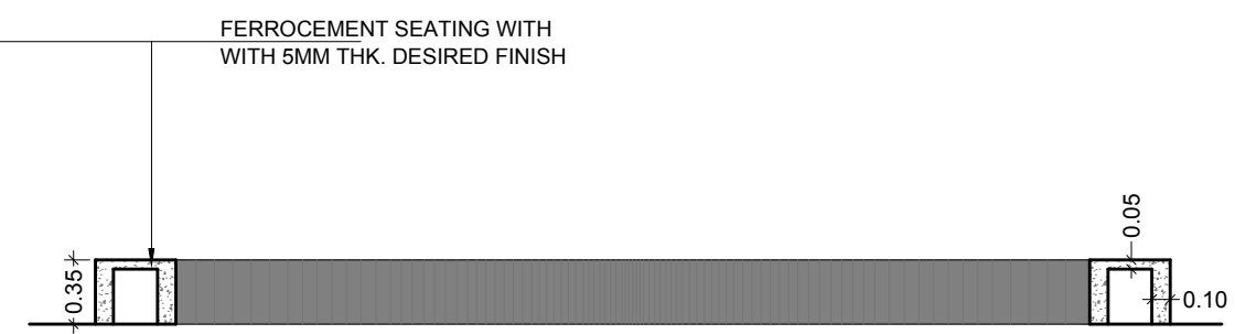
SECTION - 'A-A' (TYP.) (SCALE : 1:50)
