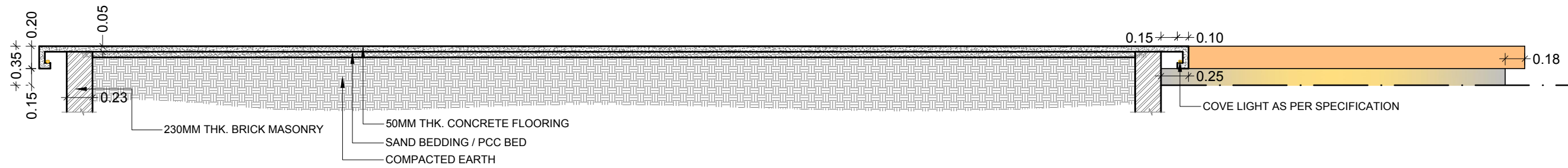
SECTION - 'A-A' (TYP.) (SCALE : 1:50)
