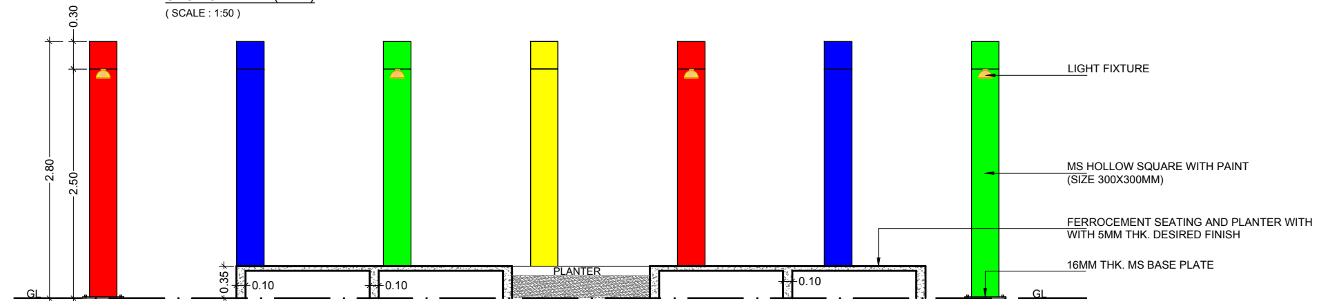
SECTION - 'A-A' (TYP.) (SCALE : 1:50)
